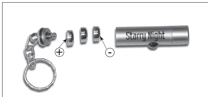
Figura 1. El lado positivo (+) de las tres pilas debe mirar hacia el extremo del llavero (o parte posterior) de la linterna y el negativo (-) debe mirar hacia el extremo del LED (o parte delantera) de la linterna.
