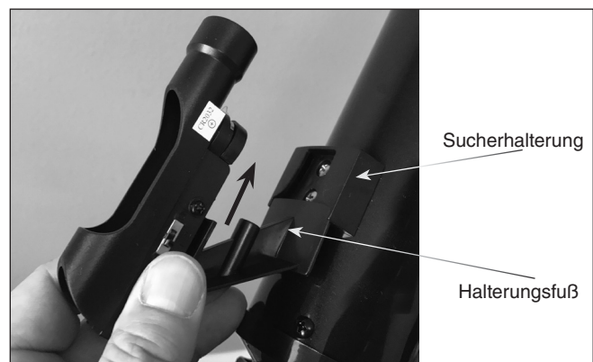
Abbildung 9. Führen Sie die Halterung des Red Dot Suchers wie gezeigt in die Basis in der Nähe des Fokussierers ein.
