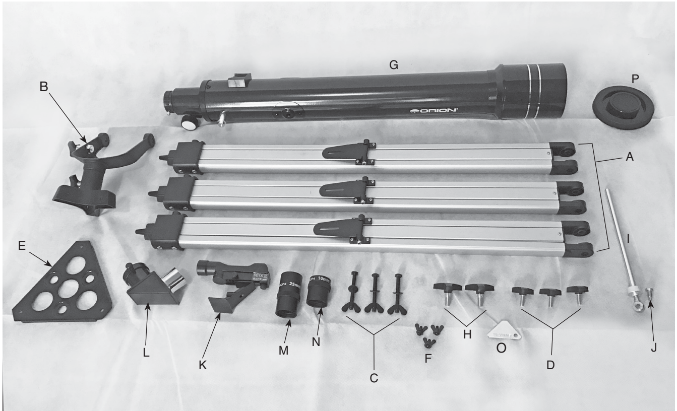
Abbildung 1. Die Teile des Observer II 70 Azimut Teleskops.
