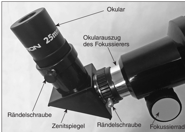
Abbildung 10. Befestigen Sie den Zenitspiegel mit der Rändelschraube im Okularauszug des Fokussierers, indem Sie die Rändelschraube der Manschette festziehen. Installieren Sie dann das Okular im Zenitspiegel.
