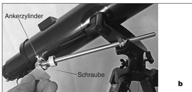
Abbildung 8. a) Schieben Sie die Stange zur Feinjustierung der Höheneinstellung durch die Metallöffnung auf der Gabelmontierung. b) Befestigen Sie das andere Ende der Stange am Ankerzylinder auf dem Optiktrohr.
