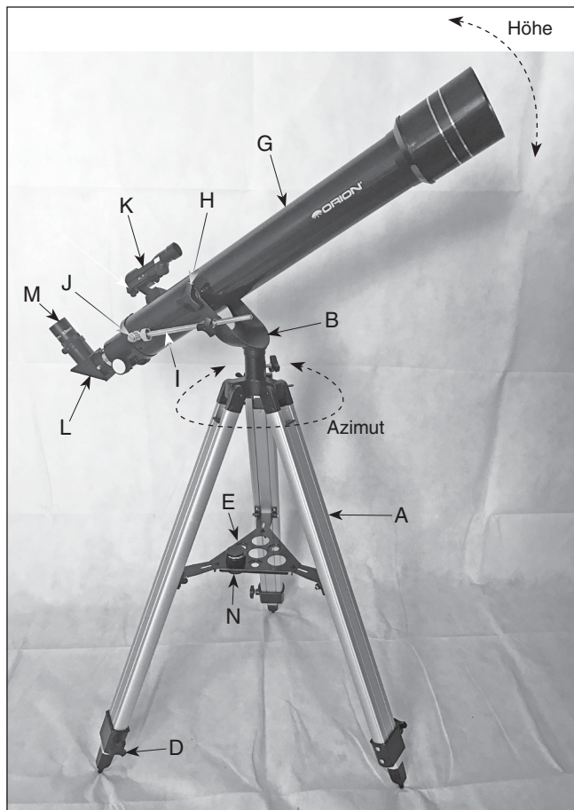
Abbildung 2. Das Observer II 70 Azimut-Refraktoreleskop vollständig montiert, mit Bezeichnung der wichtigsten Teile
