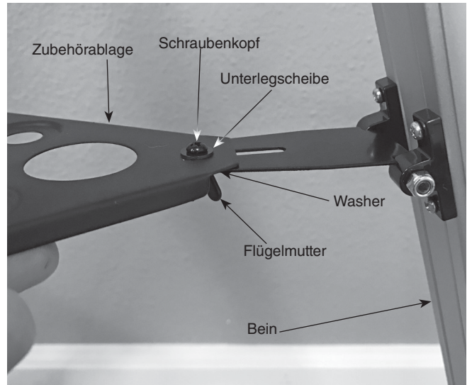
Abbildung 5. Befestigen Sie die Zubehörablage mithilfe der mitgelieferten Teile an den Halterungen der drei Beinstreben.
