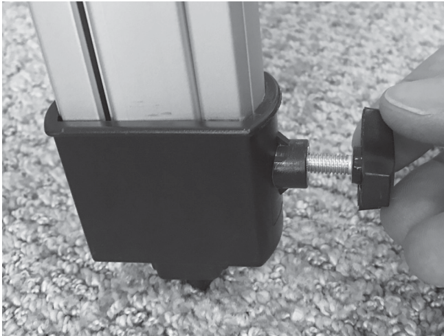
Abbildung 4. Schrauben Sie eine Rändelschraube für die Stativbeinarretierung in jedes der Beine. Seien Sie dabei vorsichtig und ziehen Sie die Schraube nicht zu fest.
