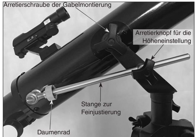
Abbildung 12. Die Stange zur Feinjustierung und das Daumenrad ermöglichen eine feinjustierte Höhenkontrolle.
