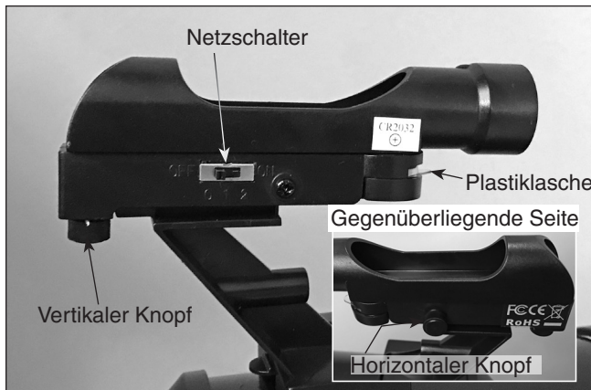
Abbildung 11. Der Red Dot Sucher verfügt über vertikale und (eingesetzte) horizontale Einstellknöpfe für die Ausrichtung mit dem Teleskop.
