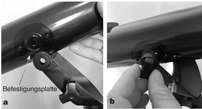
Abbildung 7. a) Platzieren Sie das Optiktrohr in der Gabelmontierung, wobei die Bohrungen der Befestigungsplatten auf denen der Gabelmontierung liegen müssen. b) Schrauben Sie die Arretierschraube der Gabelmontierung in die Gewindebohrungen der Befestigungsplatten.
