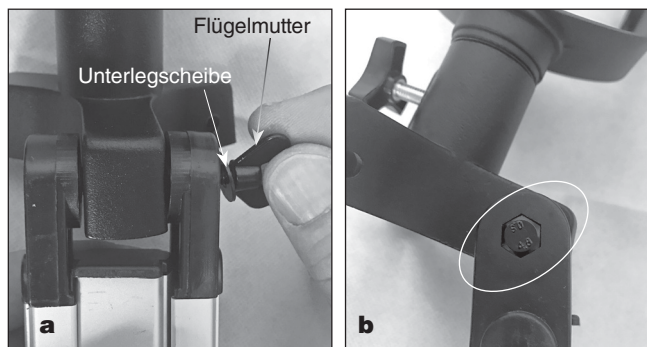
Abbildung 3. a) Befestigen Sie die drei Stativbeine an der Montageplattform, b) sorgen Sie dafür, dass der Sechskant-Bolzenkopf in der sechseckigen Aussparung des Stativbeins platziert ist.
